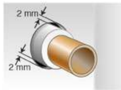
Hålfogning för rör genomföringar i vägg eller golv med tätskikt.
