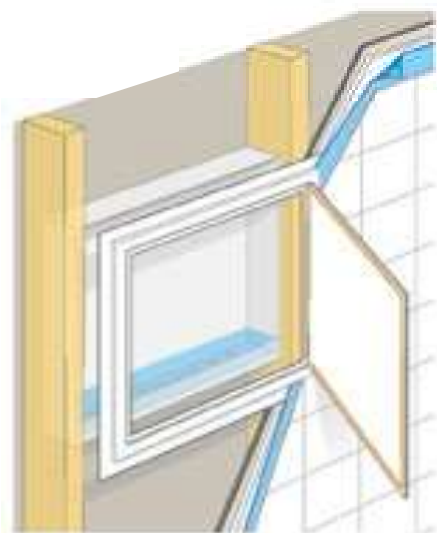
Exempel på serviceöppning: fördelarskåp med vattentät lucka och ram.
