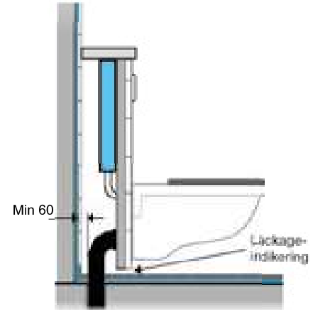
Tätskikt bakom WC med inbyggd spolcistern i våtrum.
