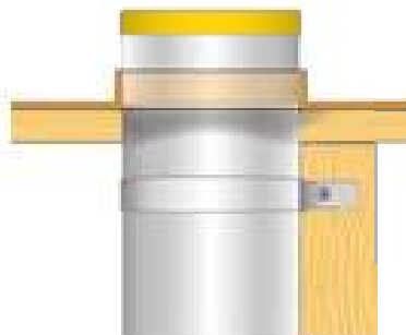
Fixering i trä.
