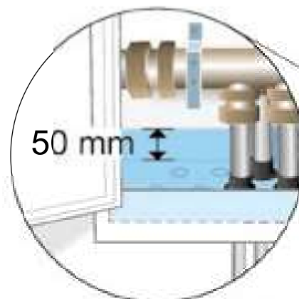
Prefabricerad konstruktion, exempelvis fördelarskåp. Rörgenomföringar genom botten ska vara vattentäta.
