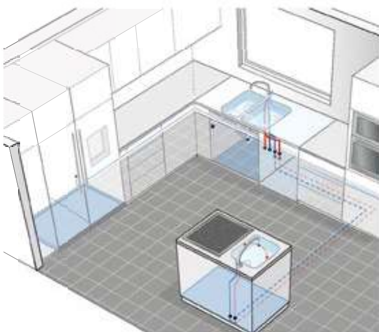
Exempel på vattentäta underlag.
