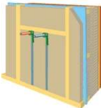
Exempel på rörförläggning på "varma sidan" av isolering i yttervägg.
