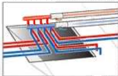
Fördelarrör i rum med vattentätt golv
