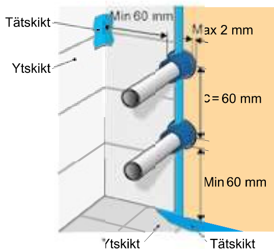
Rör genomföring i vägg med tätskikt för rör upp till 32 mm.
