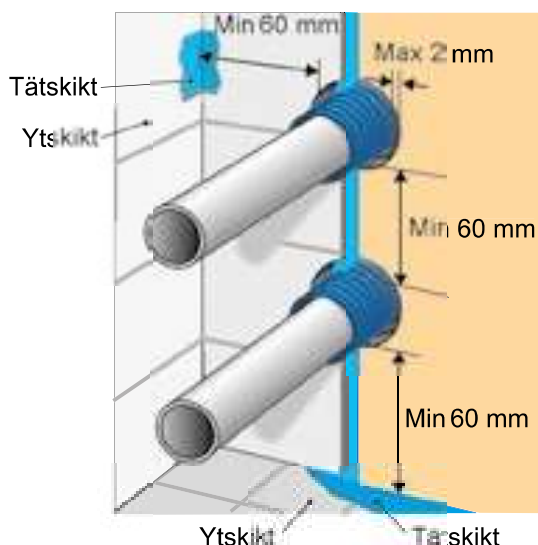
Rör genomföring i vägg med tätskikt för rör över 32 mm.
