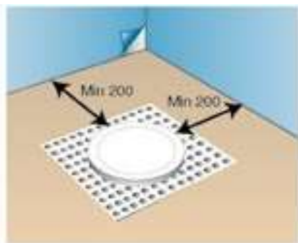
Golvbrunn i våtrum.
