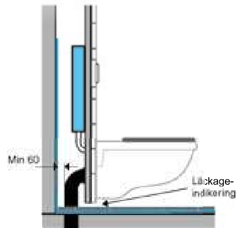
Tätskikt bakom WC med inbyggd spolcistern i WC-rum.
