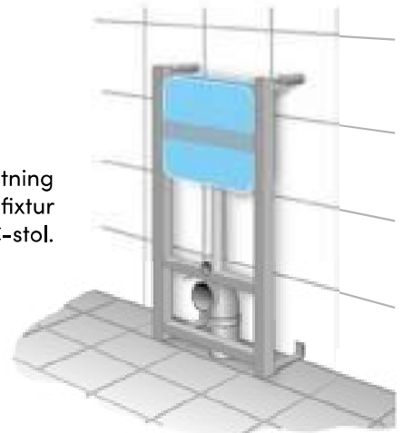
Tätskikt bakom WC med inbyggd spolcistern i WC-rum.
